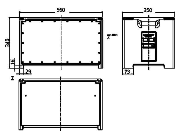
Plano 5 MB 70 Dim. en mm
