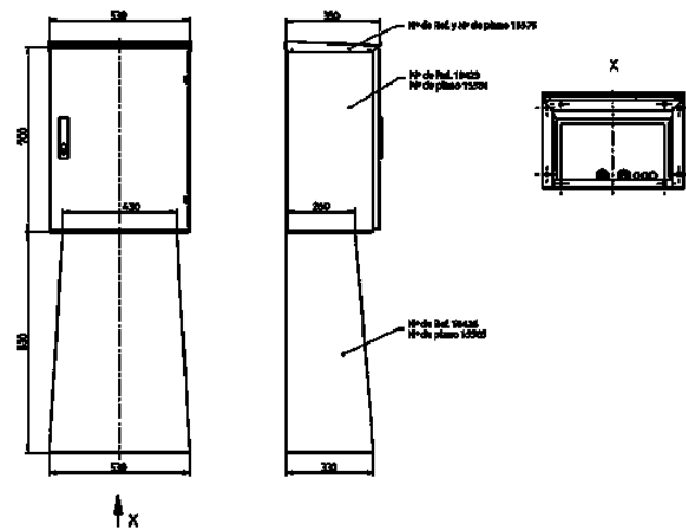
Plano 1 MB 439 Dim. en mm
